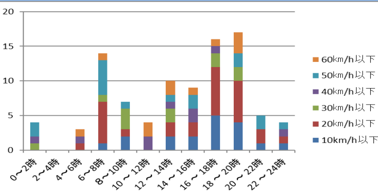
国道6号における時間帯別・危険認知速度別人身事故発生状況(過去3年)
