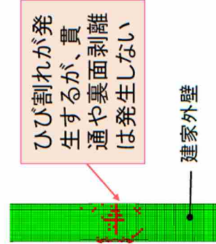
図1高放射性廃液貯蔵場(HAW)の建家外壁に対する3次元解析結果
