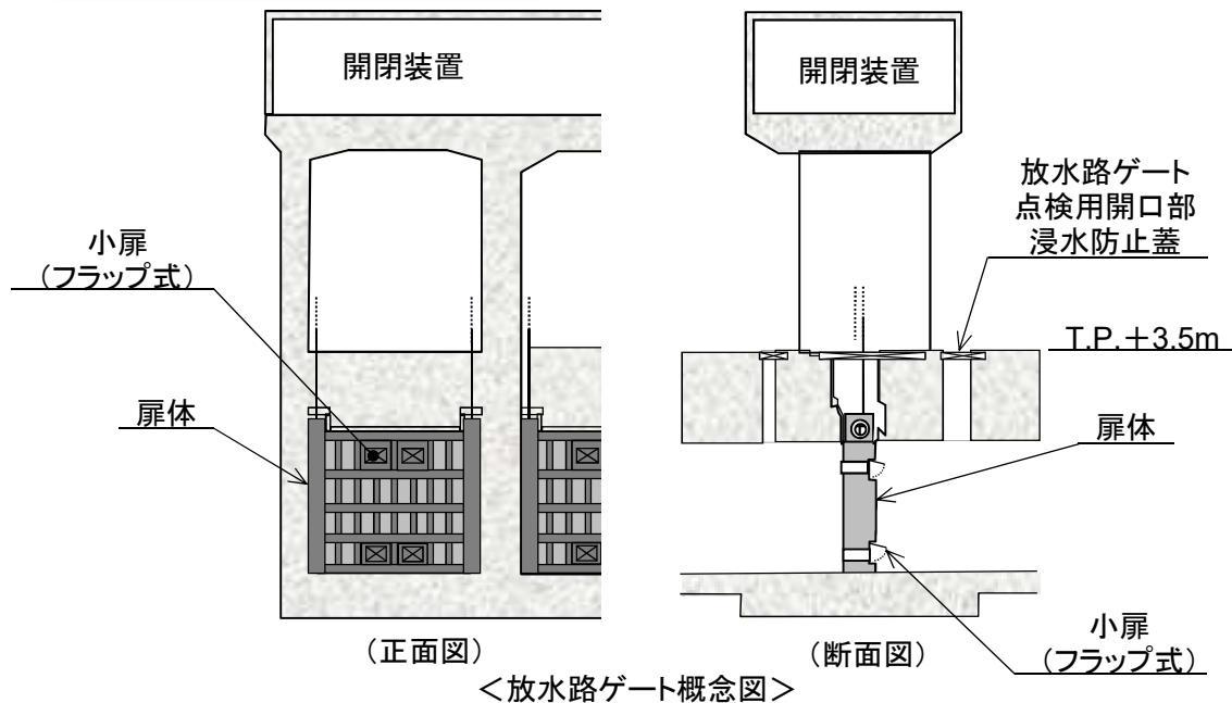
浸水防止設備(浸水防止蓋)
