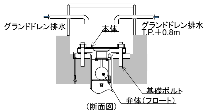
浸水防止設備(逆止弁)
