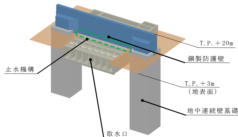
<鋼製防護壁>
