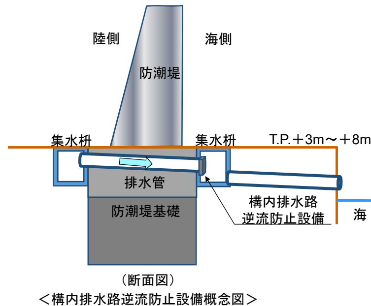
浸水防止設備(逆止弁)
