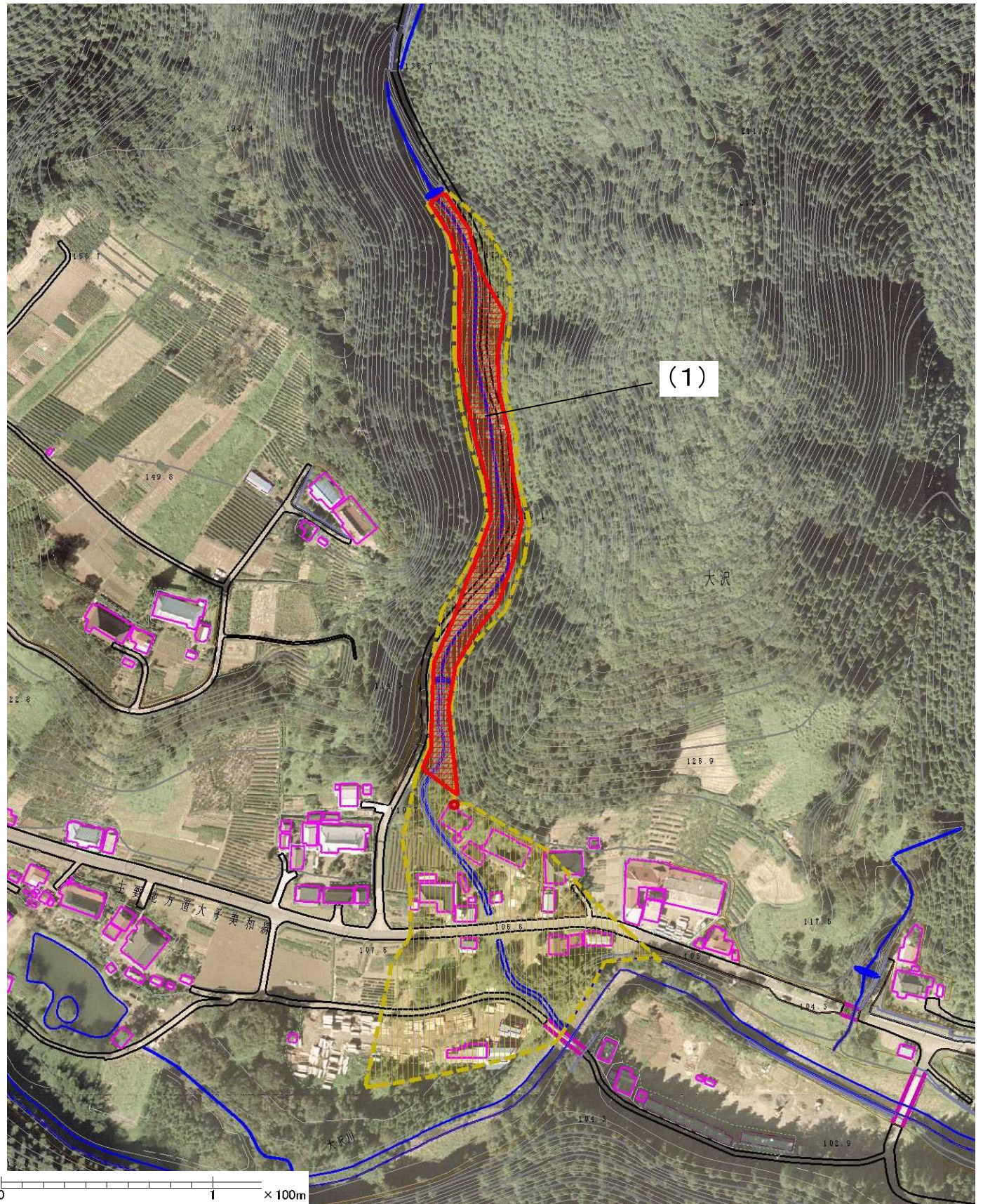
様式-2(土) 土砂災害警戒区域・土砂災害特別警戒区域区域図(その1)
