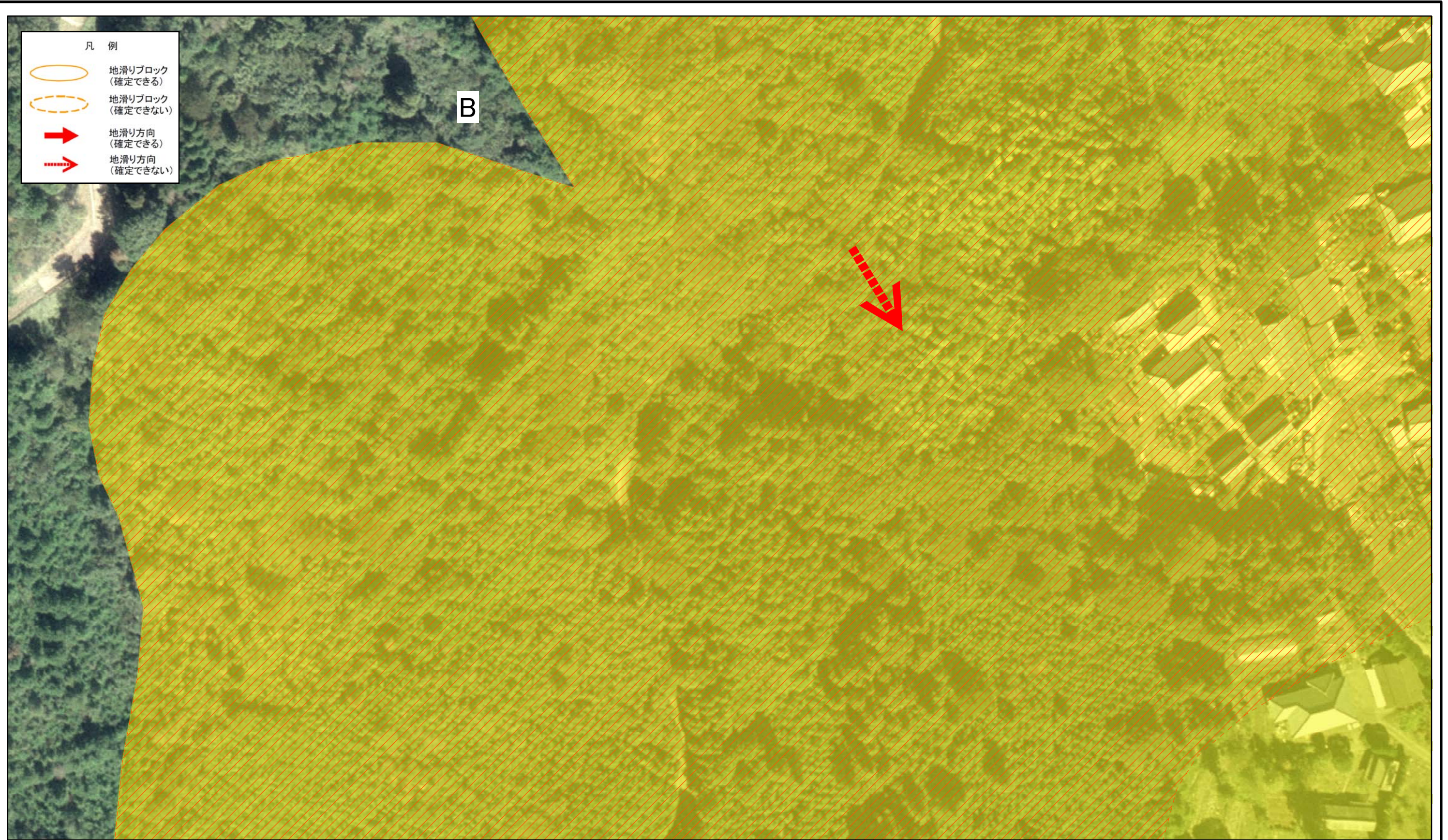
様式-3(地) 土砂災害警戒区域・土砂災害特別警戒区域 区域図
