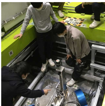
図1. iMATERIA 装置への試料取り付け作業
