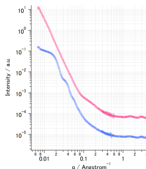
図2. シリカ粉末の SANS プロファイル（粒径100nm（赤）および30nm（青））
