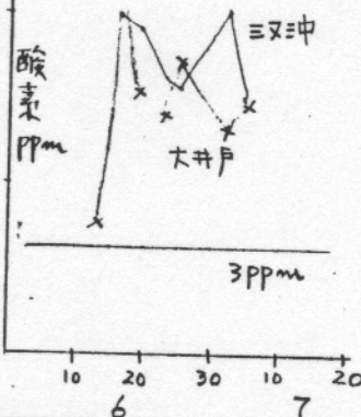
霞ヶ浦の酸素変化 (平均値)
