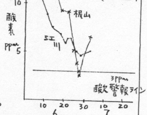
北浦の酸素変化 (平均値)
