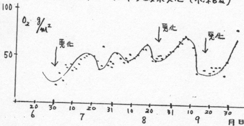
昭和54年 三又沖の酸素変化 (水深6m)
