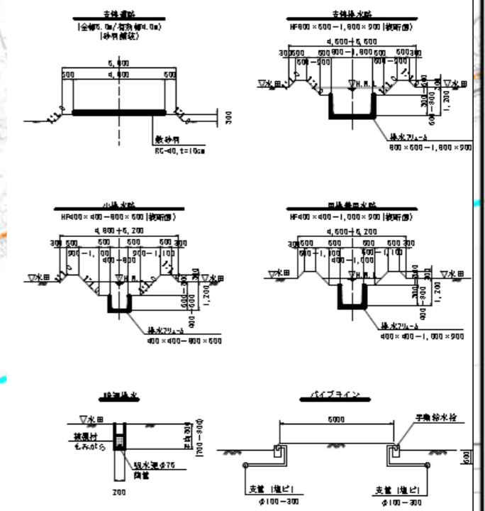
標準断面図
