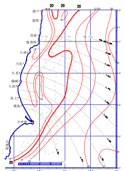
【海況図】
