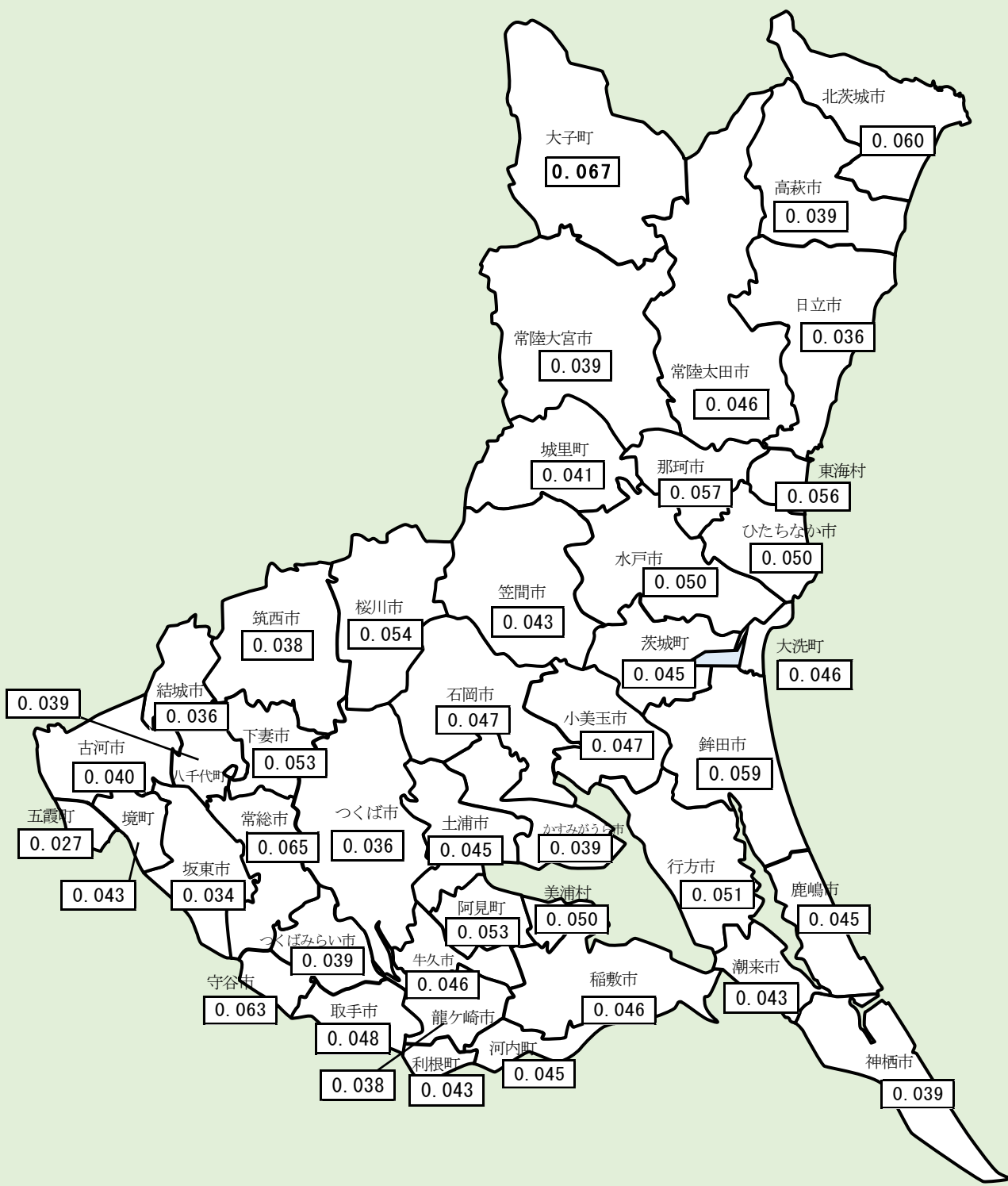
図Ⅱ-1 令和6年10月31日12時における全市町村放射線量率測定結果（地上1m） （令和6年1月31日に欠測となっている局は、直近の測定値を記載）
