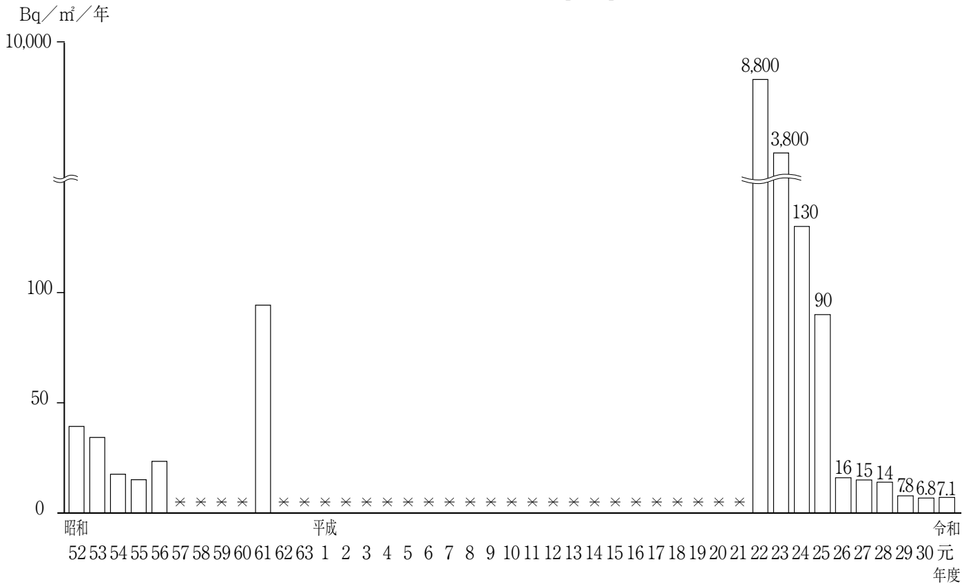
降下塵中の 137 Cs経年変化【水戸】
