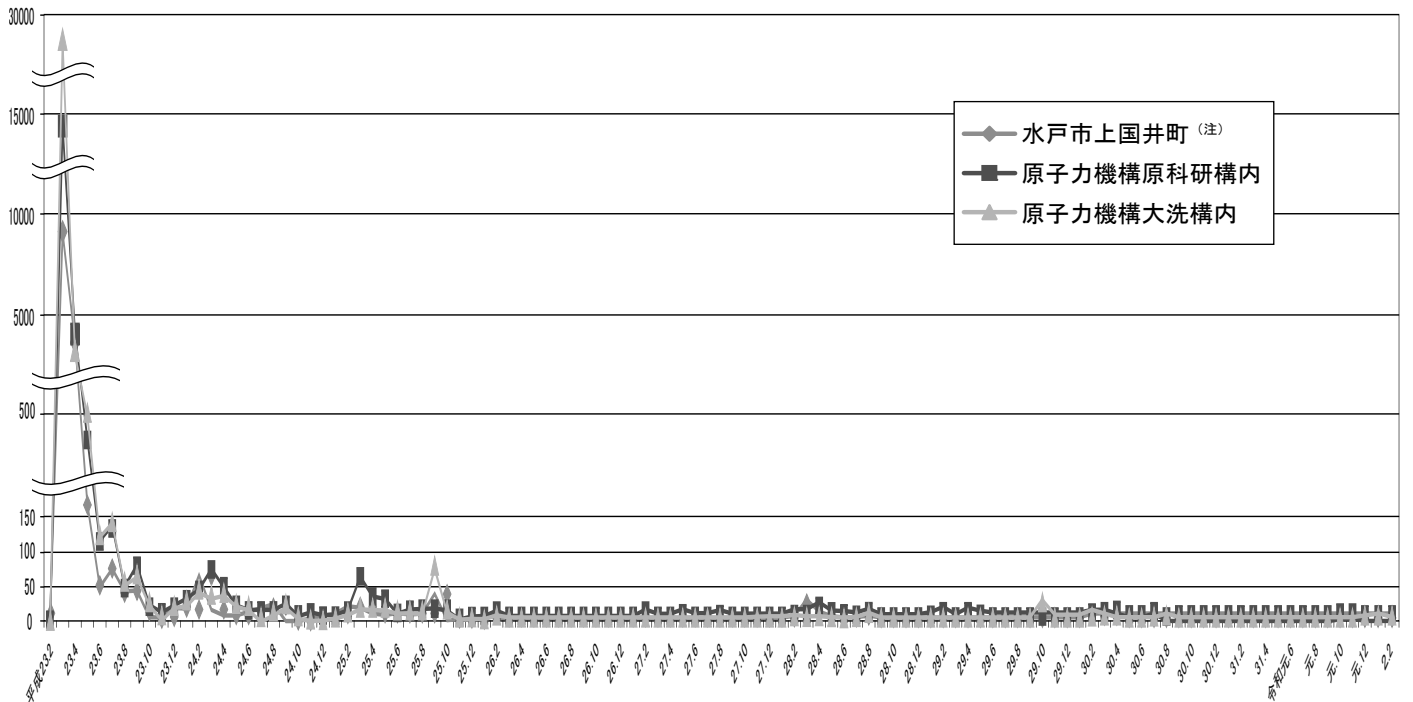
降下塵中の 137 Cs経月変化 (Bq / m 2 )
