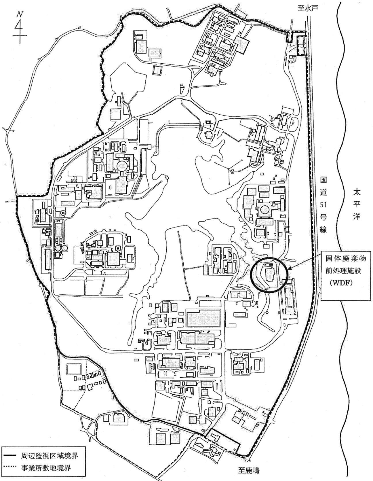
日本原子力研究開発機構 大洗研究開発センター 施設配置図
