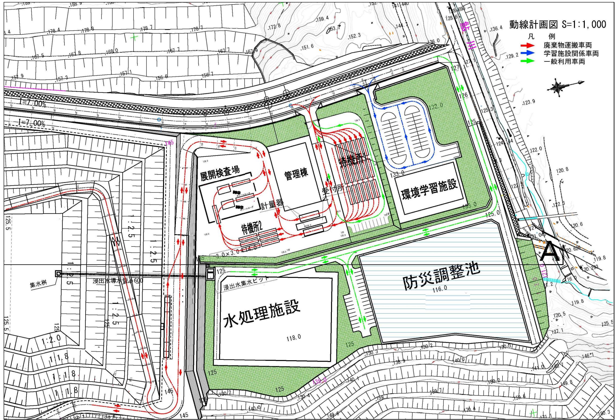
図 4.4 管理施設周辺の動線計画
