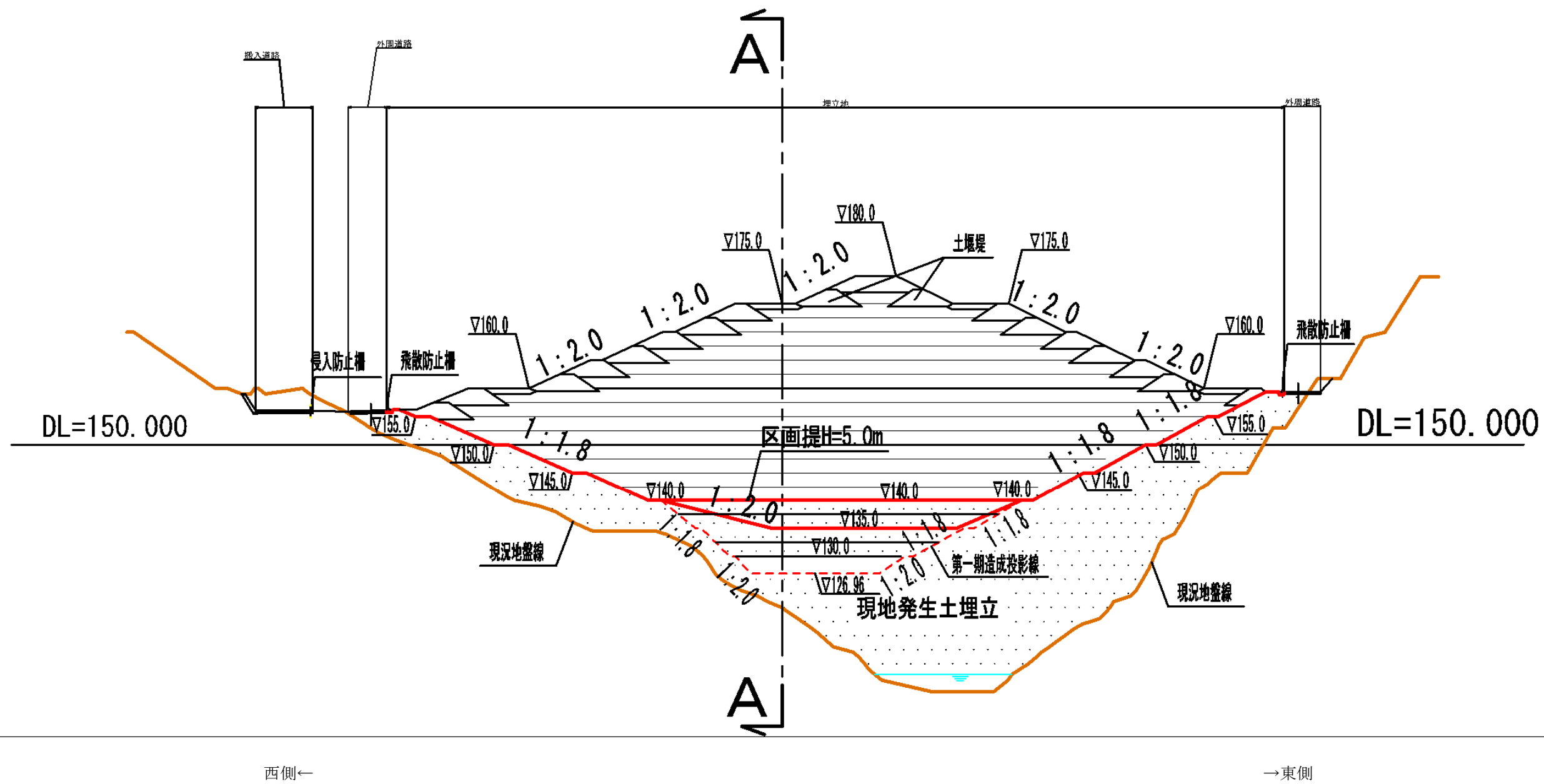
图 4.6 造成計画(横断面)
