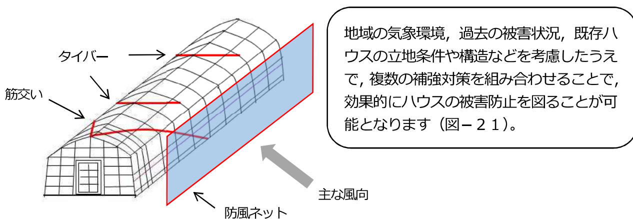
図－21 補強対策の組み合わせ例（再掲）
