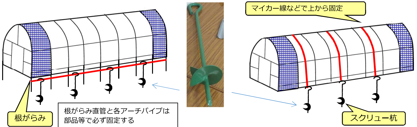
図-17 パイプハウスの基礎の強化事例
