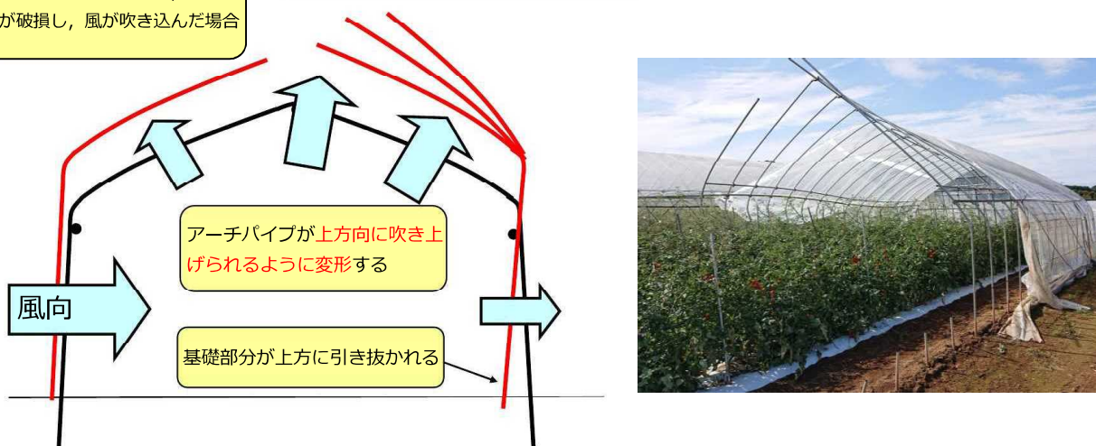
図-4 風の吹き込みにより内側から外側に破裂するパターン
