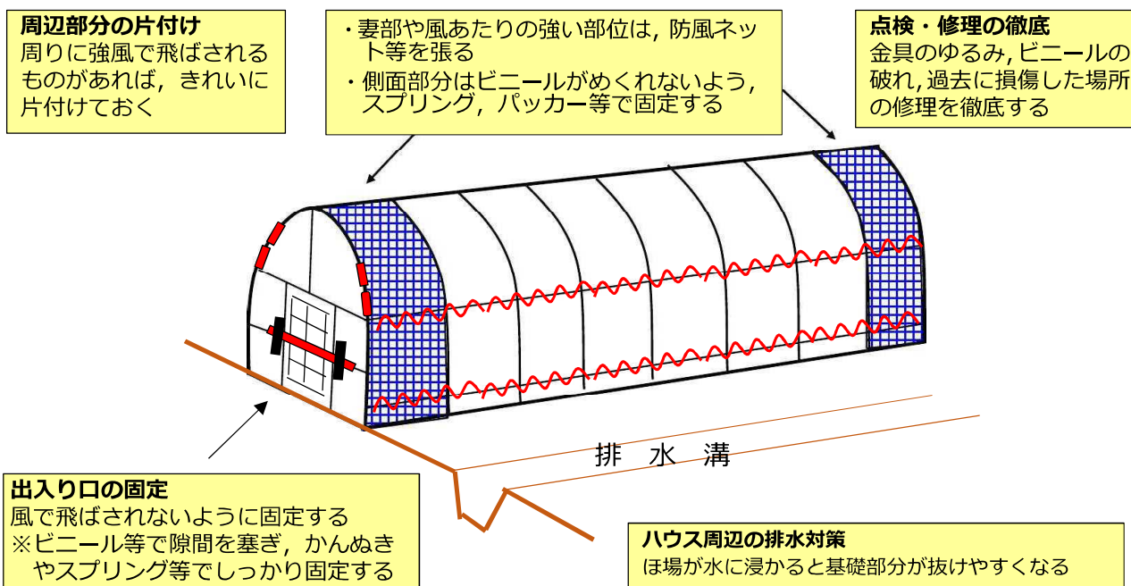
図-23 パイプハウスの強化事例
