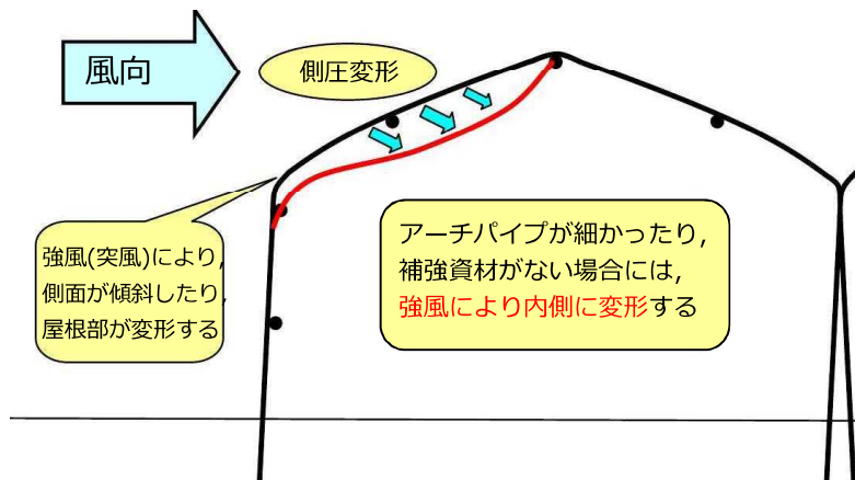
図-3 風上側の屋根部分が変形するパターン
