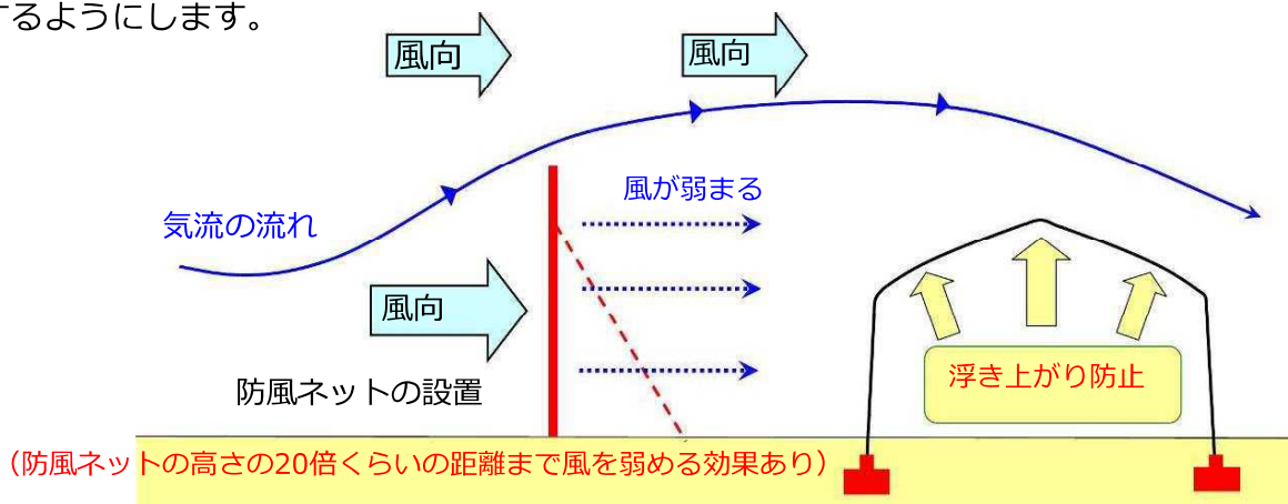
図-20 防風施設（防風ネット）の設置
